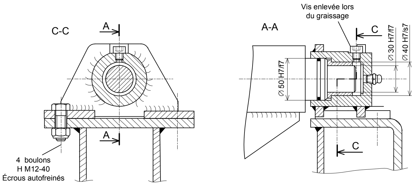
Palier de guidage du châssis intermédiaire Echelle : 0,35 (A4)
