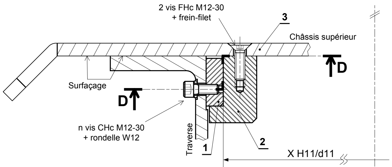
Guidage du châssis supérieur Echelle : 0,35 (A4)
